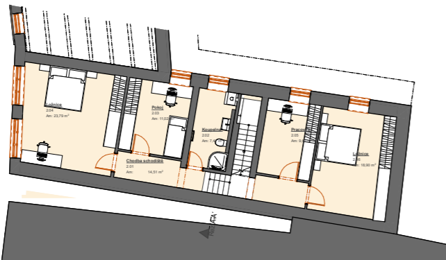
Byt č.1 Púdorys 2.NP
